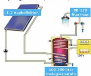
1-2 kollektoros napenergia rendszer (Szolártároló)
